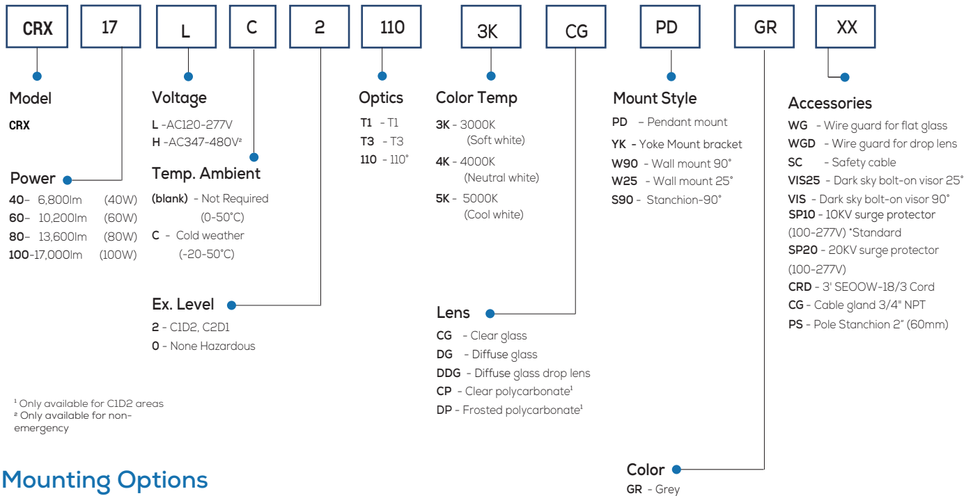
PD Pendant mount 3/4" NPT
